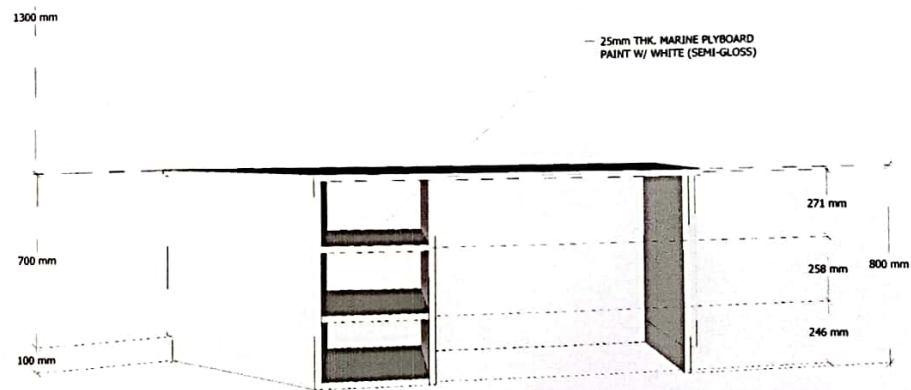
2 A.V.R. COUNTER DETAIL 2 (1 SET) A 41 SCALE:
