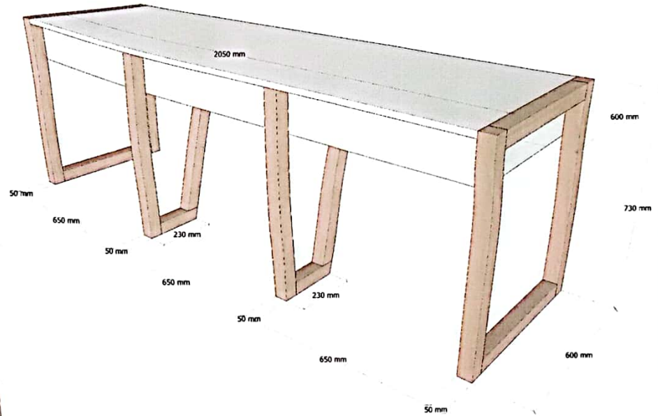
2 CLASSROOM 2 TABLE DETAIL 2 SCALE:
