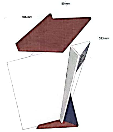
13 PODIUM DETAIL 2 (1 SET) SCALE:
