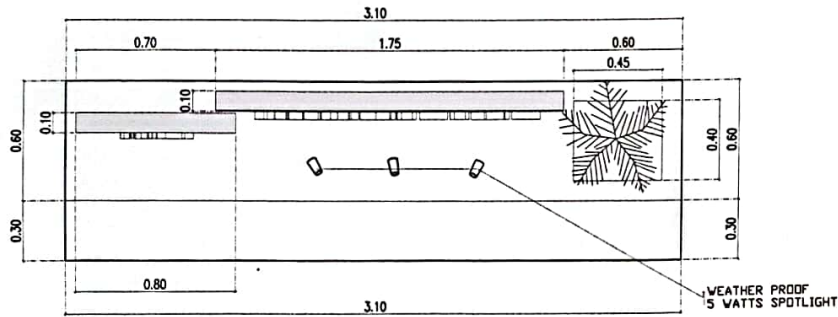
SIGNAGE TOP VIEW SCALE:
